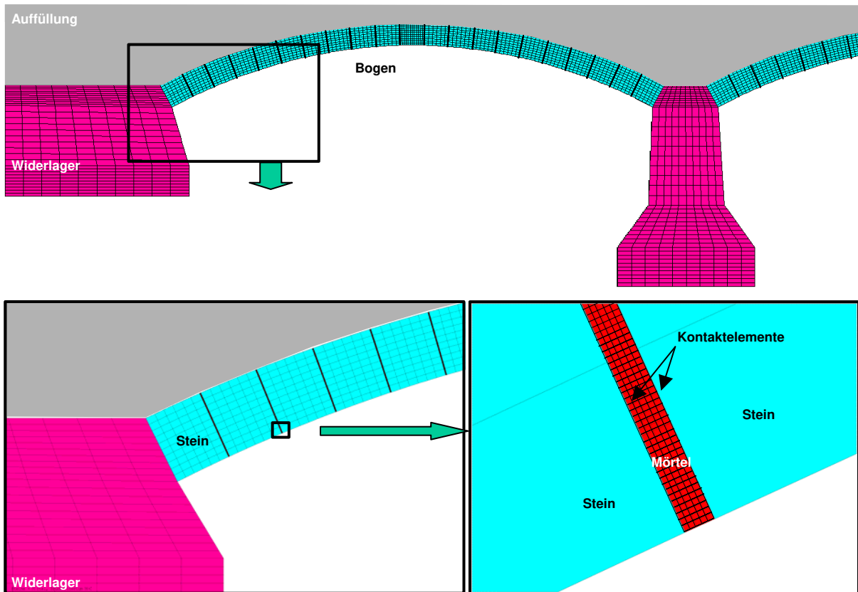
Fig. 6: FE-Vernetzung (Micromodell)
