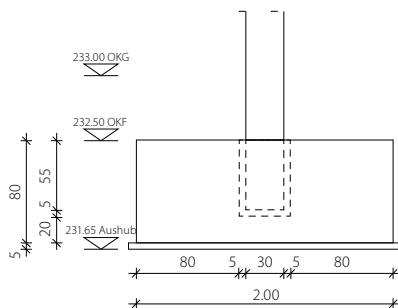
Schalplan Becherfundament mit Höhenkoten
