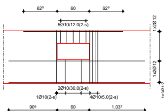
Zulagen im Öffnungsbereich
